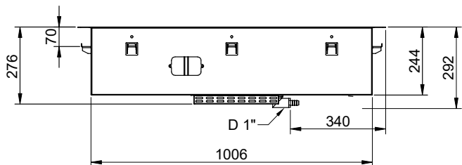
Zij aanzicht
